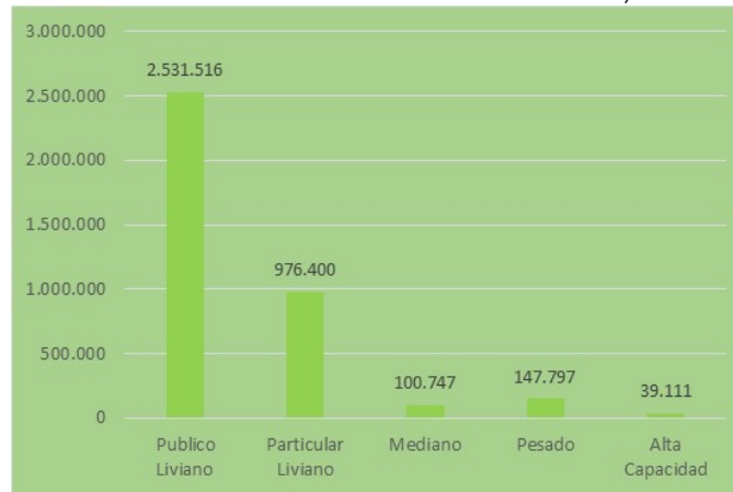
GRAFICO N° 01 LA PAZ: TRÁFICO VEHICULAR ESTACIÓN AUTOPISTA, ENERO – JUNIO 2018
